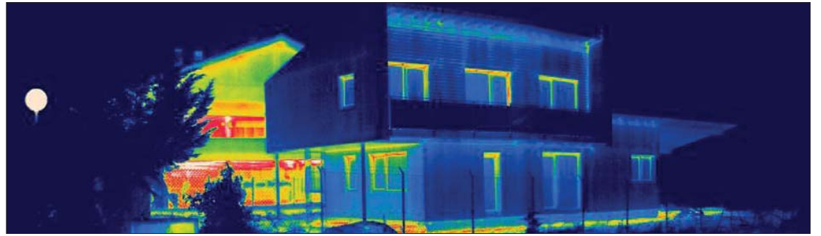
Imagen termográfica de un edificio bien aislado delante y detrás un edificio de construcción convencional con escaso aislamiento. Las fugas de calor son evidenciadas por colores cálidos. Imagen Google.
